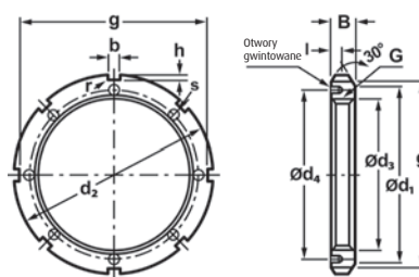
Nakrętka z podkładką kształtową od AN44/HM44T
